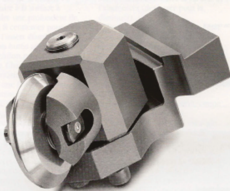
UBT-T Brunissoir type porte-outil indexable
